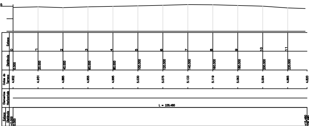
PERFIL LONGITUDINAL ESC. V: 1/1000 ESC. H: 1/100
