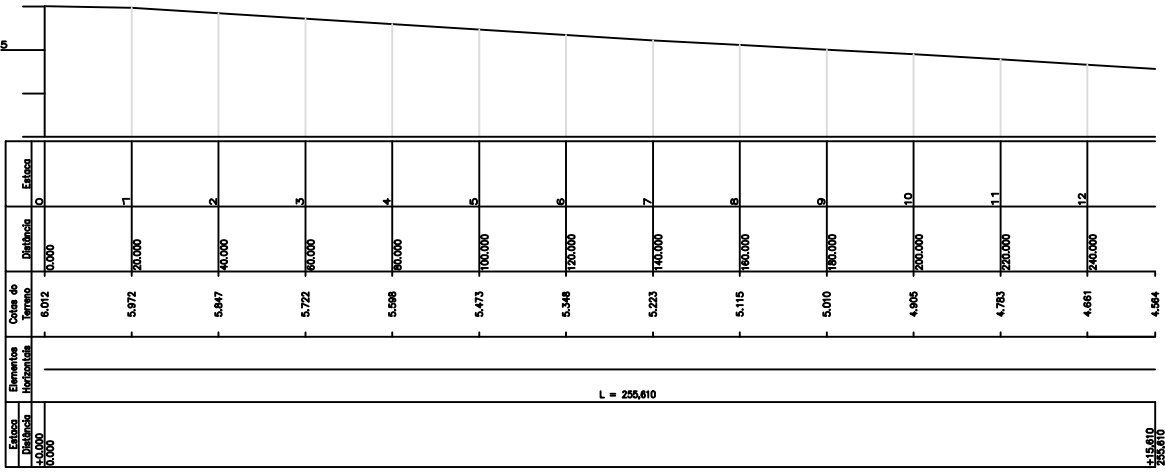
PERFIL LONGITUDINAL ESC. V: 1/1000 ESC. H: 1/100
