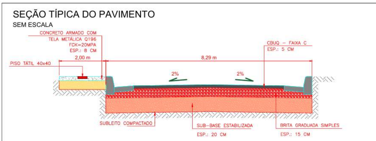
Figura 01: Seção do pavimento.
