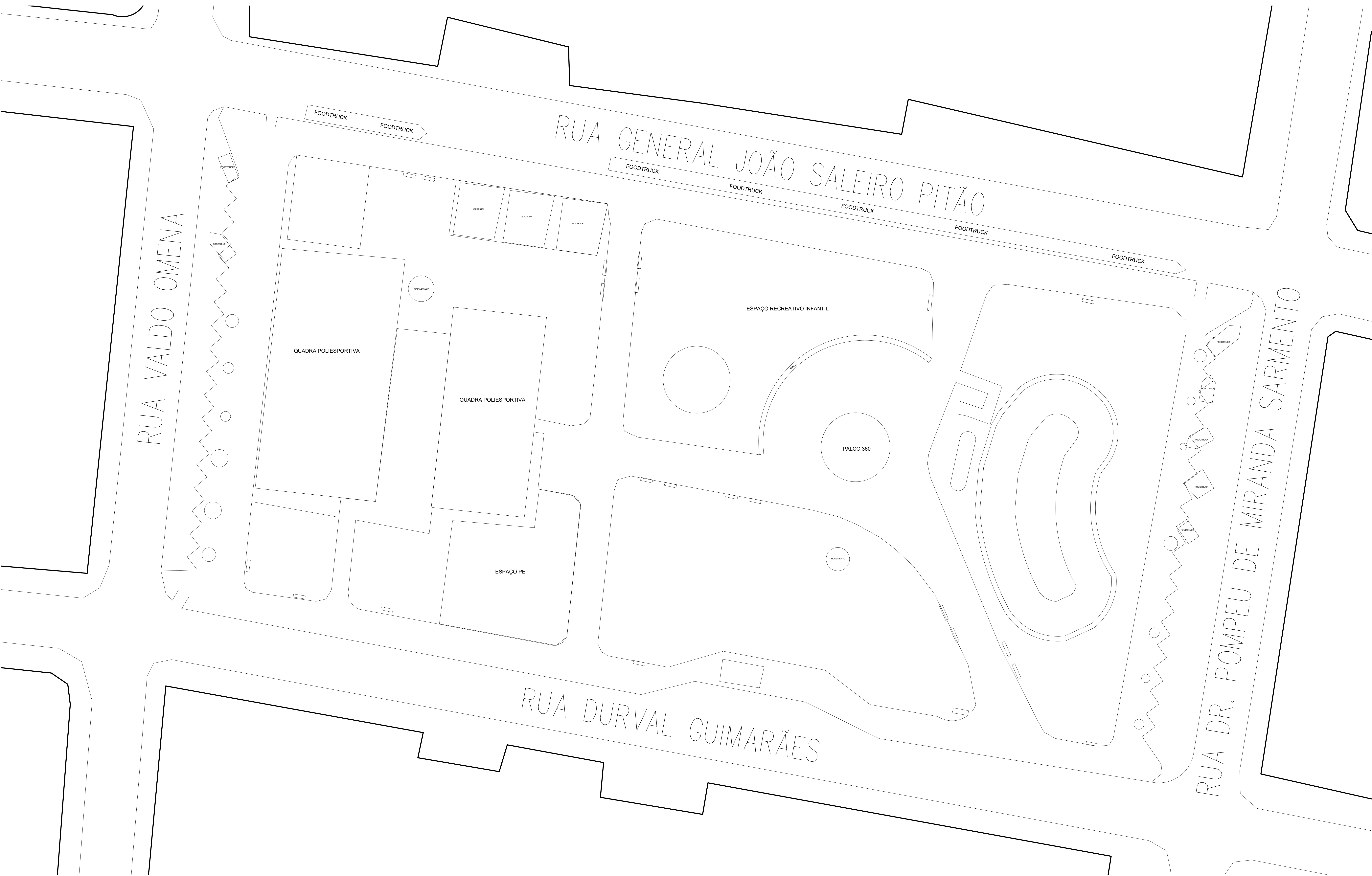
01 PLANTA BAIXA DE LEVANTAMENTO ESCALA 1/200
