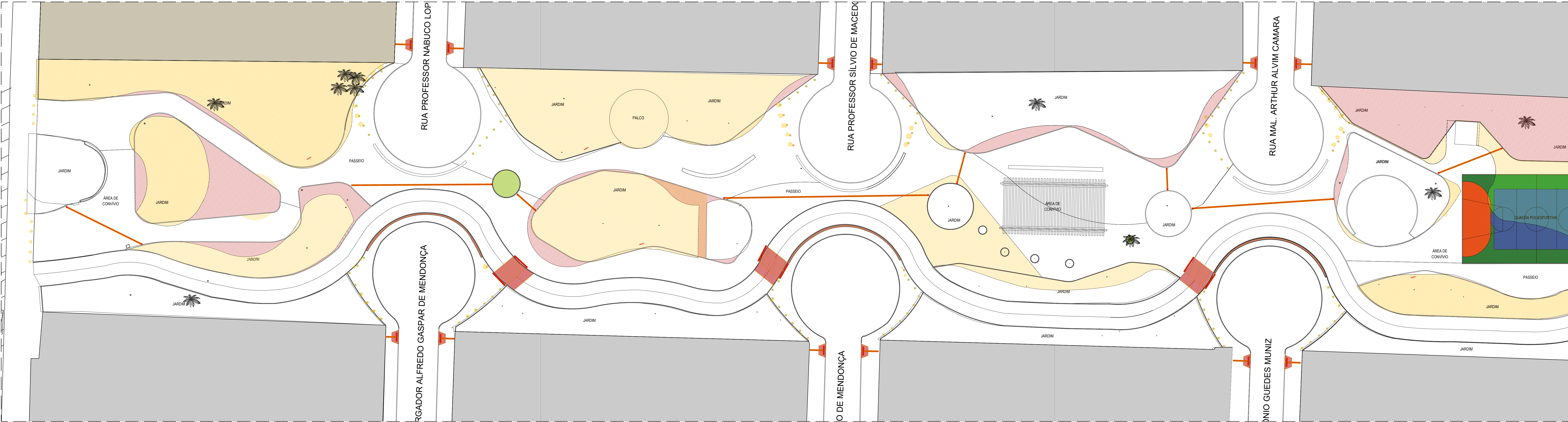
4 PLANTA DEMOLIR/CONSTRUIR - TRECHO 01 ESC.: 1/250
