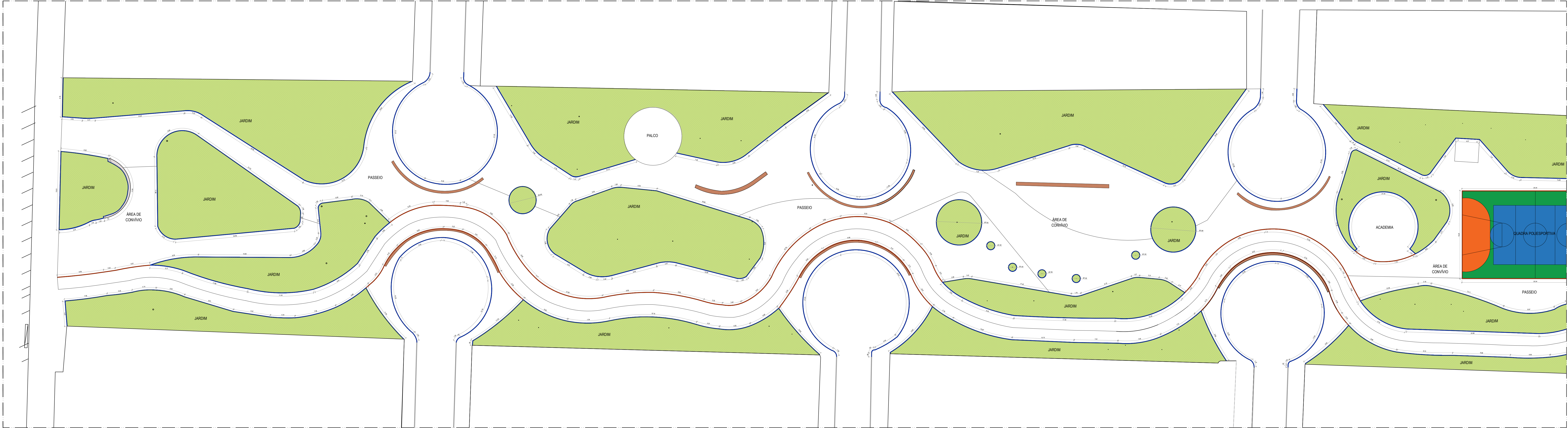
12 PLANTA DE MEIO FIO - TRECHO 01 Escala: 1/250
