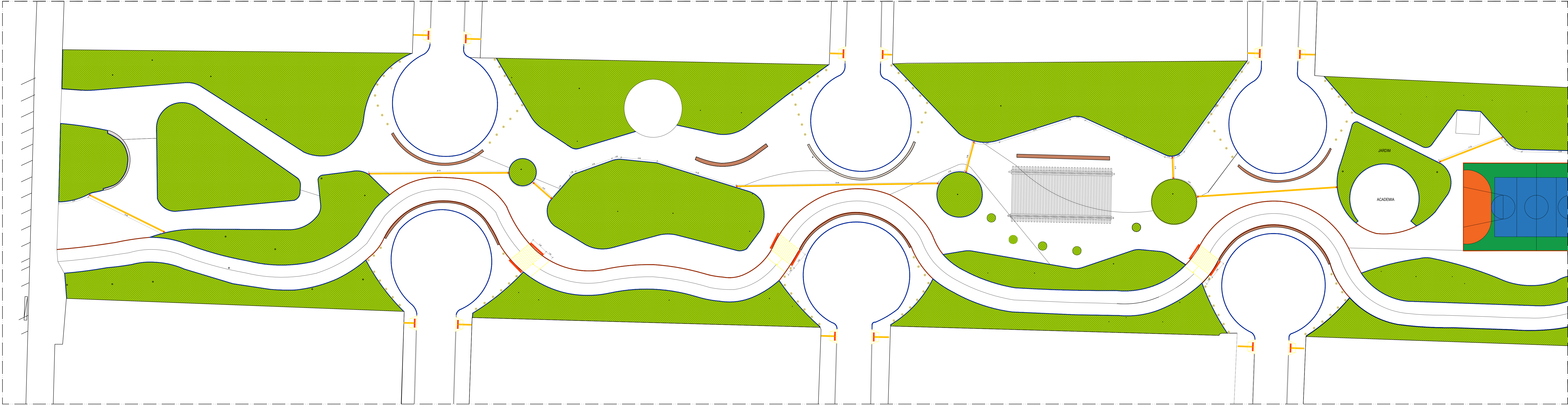
16 PLANTA DE ACESSIBILIDADE - TRECHO 01 ESC.: 1/250
