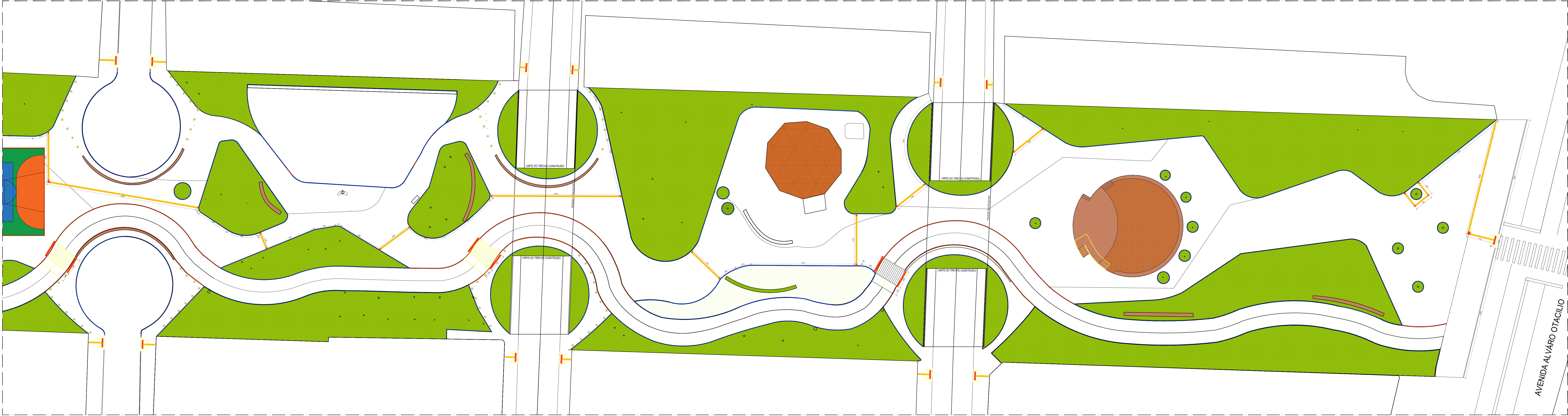
17 PLANTA DE ACESSIBILIDADE - TRECHO 02 ESC.: 1/250
