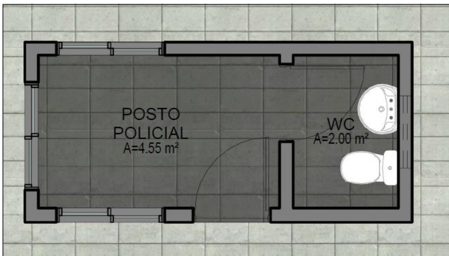
Imagem 09: Planta Baixa Pav. Térreo Edificação de Apoio – Posto Policial.
