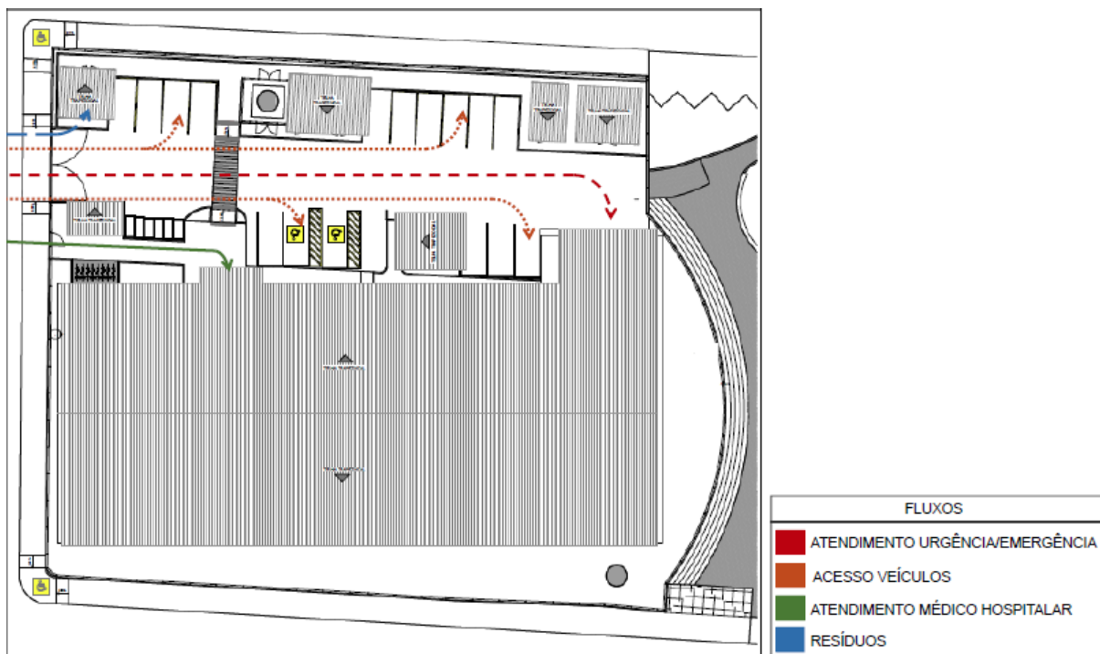
Imagem 04: Esquema dos fluxos da UPA Jacintinho.
