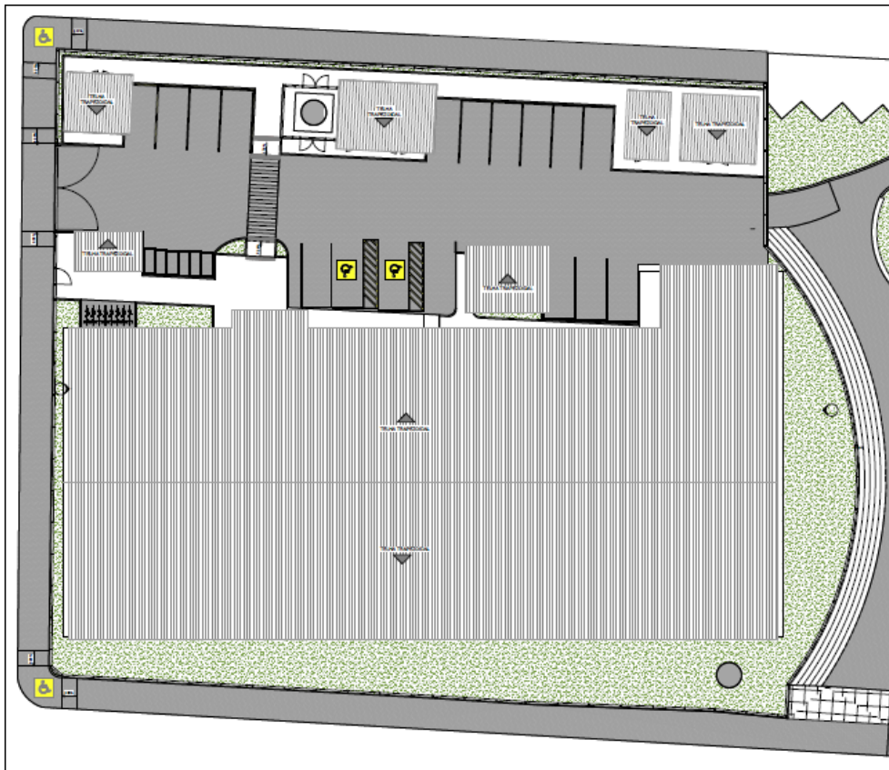
Imagem 02: Implantação da UPA Jacintinho.
