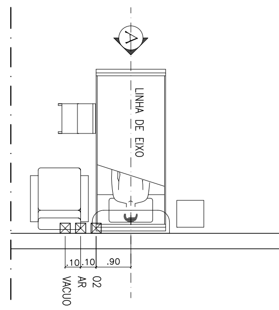
PLANTA BAIXA - PONTO DE GASES ESCALA 1/50
