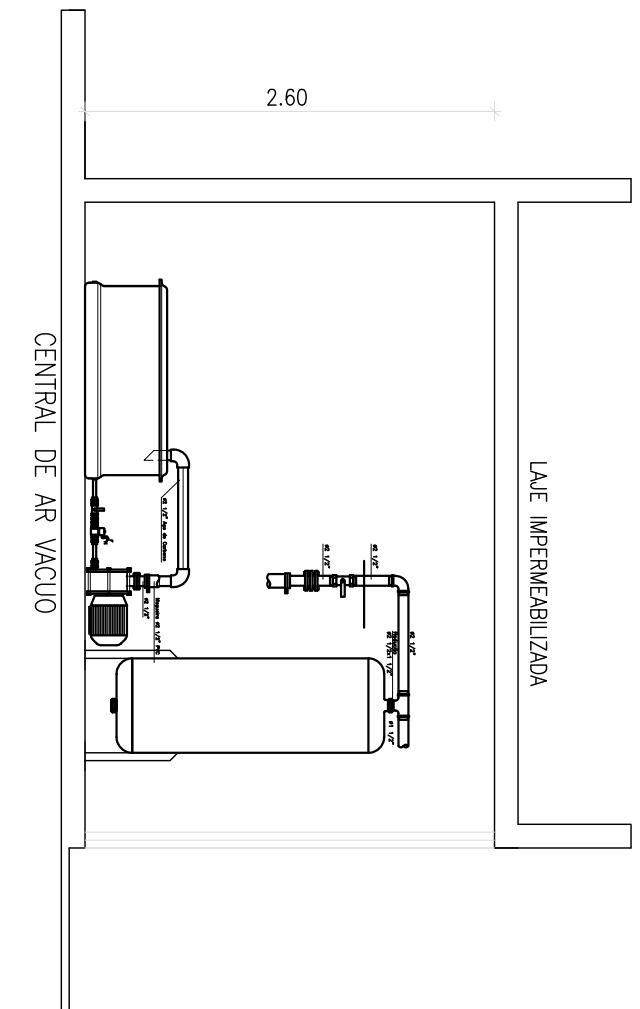
CORTE D-D' ESCALA 1/50
