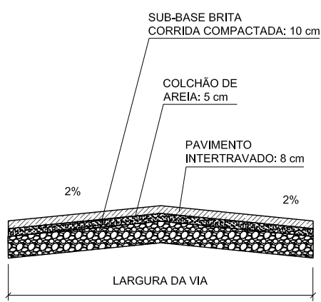
DETALHE 2: VIA DE ACESSO SEM ESCALA
