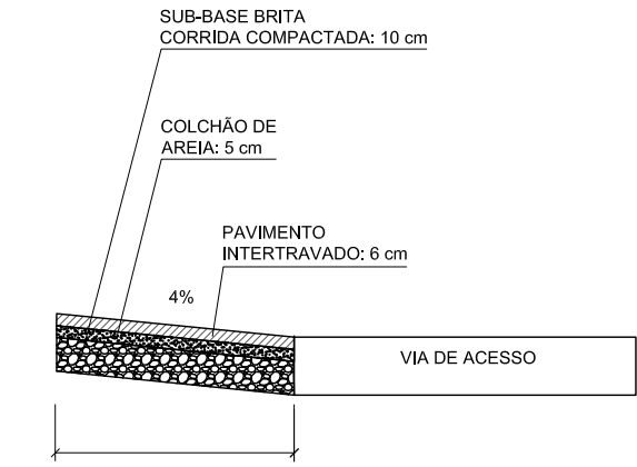
DETALHE 1: ESTACIONAMENTO SEM ESCALA
