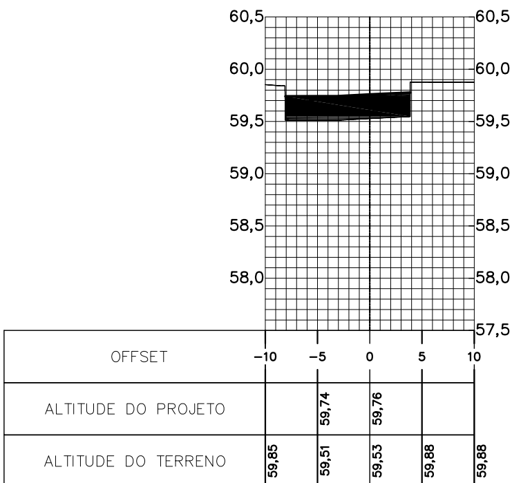
Perfil Longitudinal - 0+34,65 Escala: H(1:500); V(1:50)
