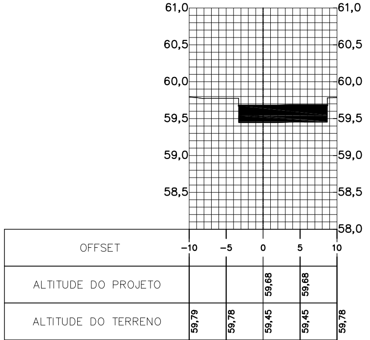
Perfil Longitudinal - 0+21,50 Escala: H(1:500); V(1:50)
