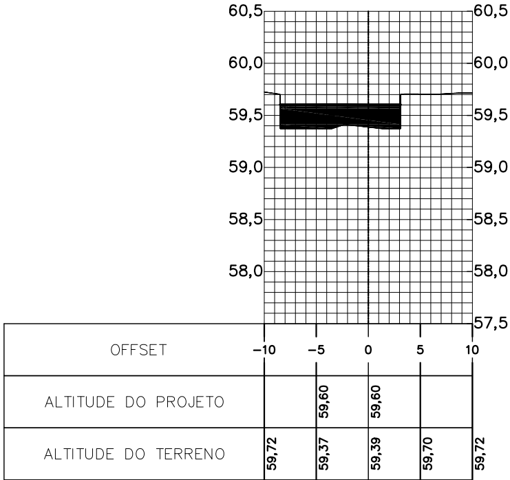
Perfil Longitudinal - 0+6,96 Escala: H(1:500); V(1:50)
