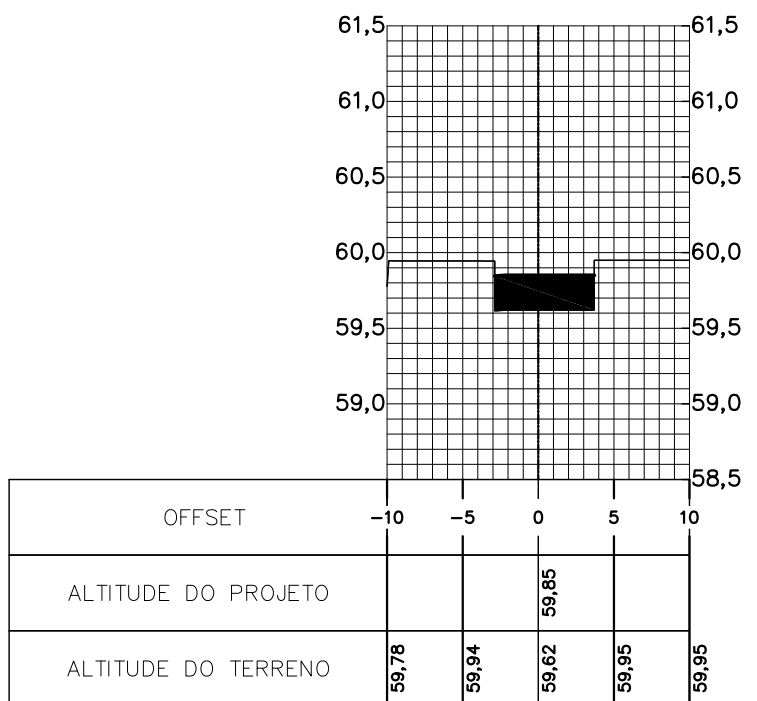
Perfil Longitudinal - 0+55,15 Escala: H(1:500); V(1:50)
