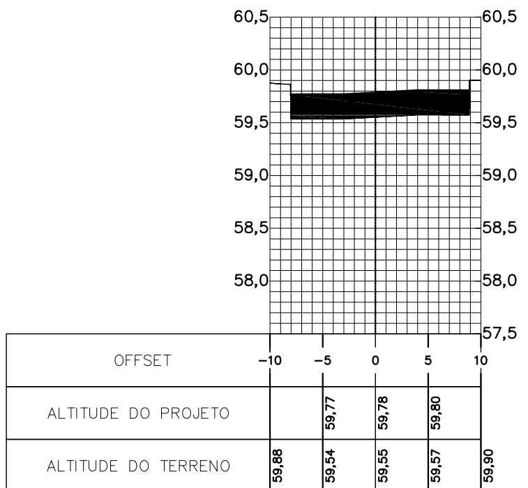
Perfil Longitudinal - 0+39,51 Escala: H(1:500); V(1:50)
