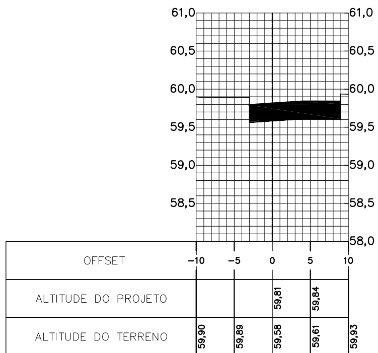
Perfil Longitudinal - 0+44,58 Escala: H(1:500); V(1:50)
