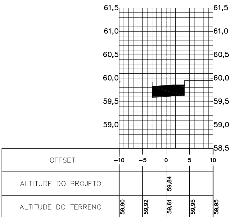
Perfil Longitudinal - 0+50,00 Escala: H(1:500); V(1:50)
