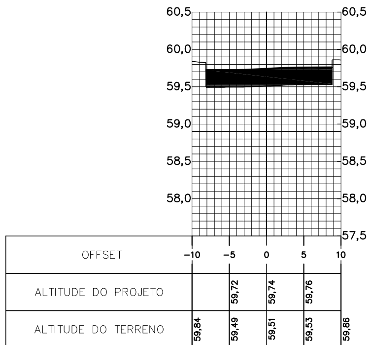
Perfil Longitudinal - 0+31,40 Escala: H(1:500); V(1:50)
