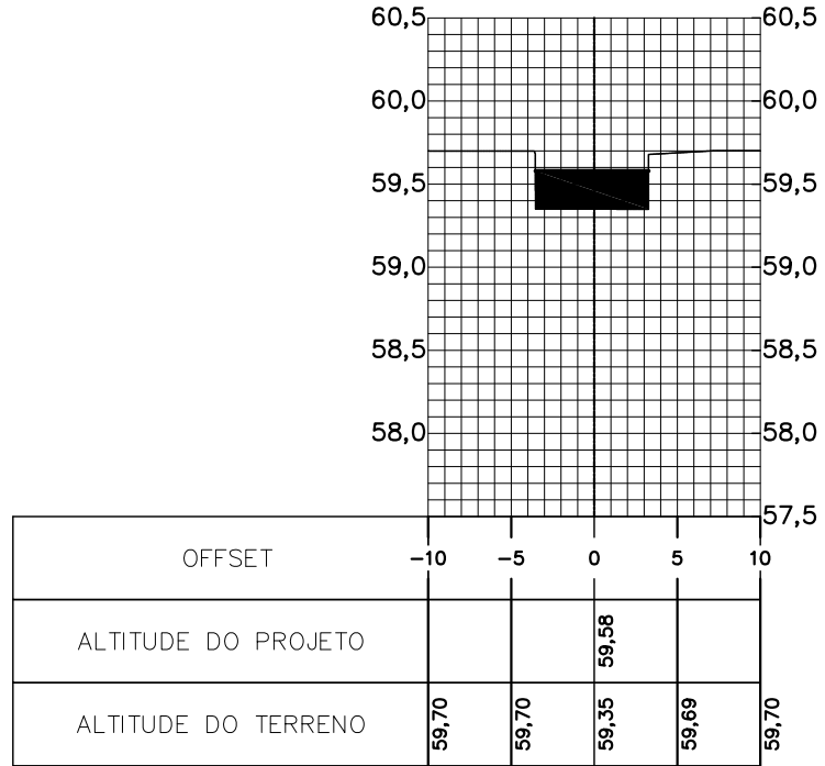
Perfil Longitudinal - 0+2,20 Escala: H(1:500); V(1:50)
